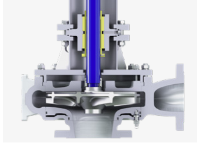
无堵塞涡流叶轮, 用于含有大颗粒的介质
