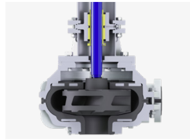
闭式叶轮 (橡胶衬里) 用于泥浆工况
