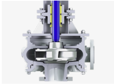
闭式叶轮用于泥浆工况
