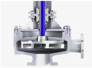
Vortex 叶轮用于泥浆工况
