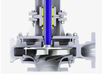
开式叶轮, 用于清洁和轻微污染的介质
