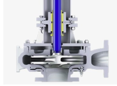
耐磨叶轮用于磨蚀性介质
